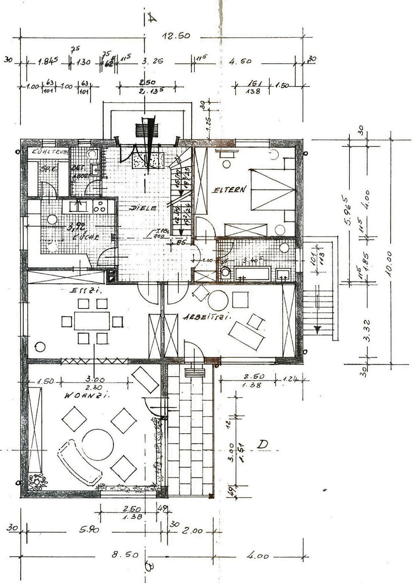
ERDGESCHOSS
